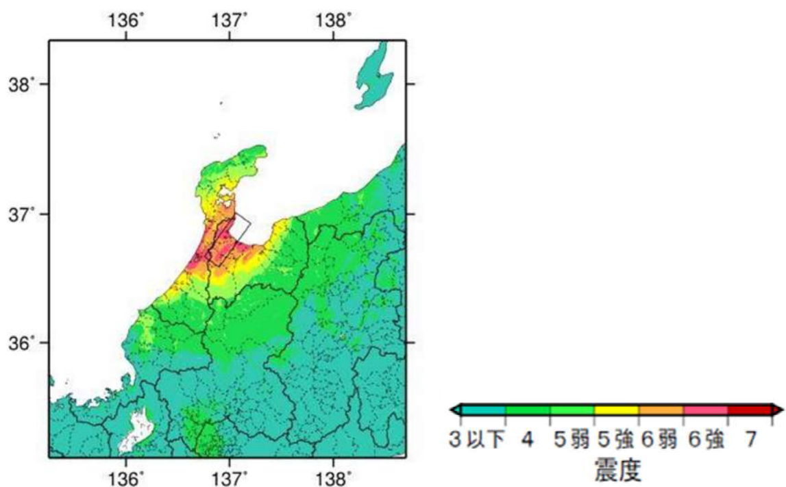
簡便法震度分布
