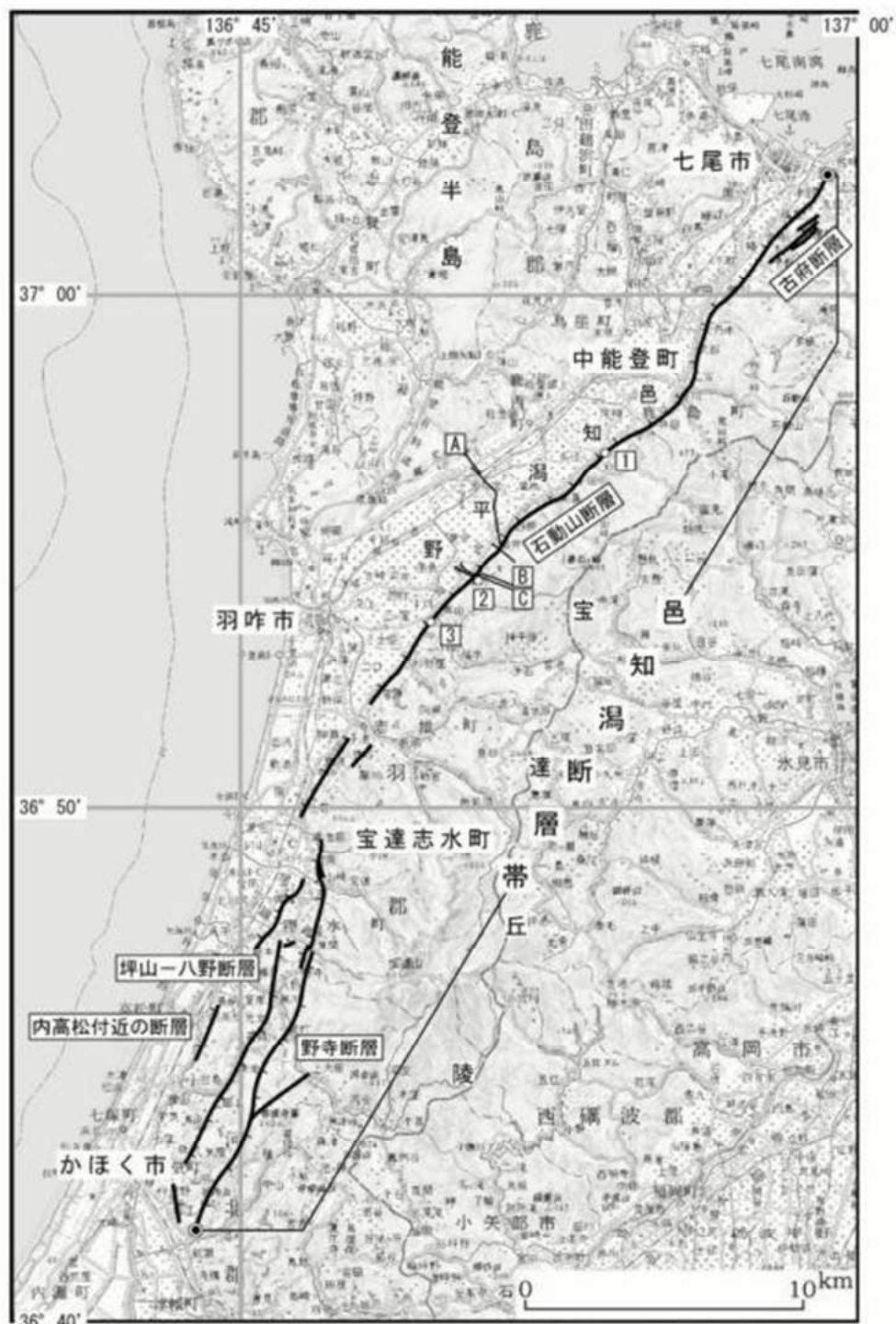
図2 邑知潟断層帯の位置と主な調査地点
