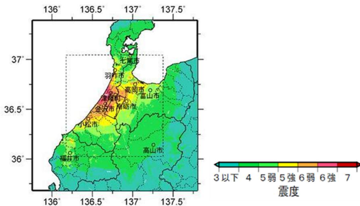
簡便法震度分布
