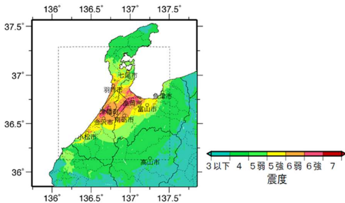
簡便法震度分布
