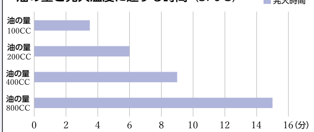
油の量と発火温度に達する時間 (370℃)
